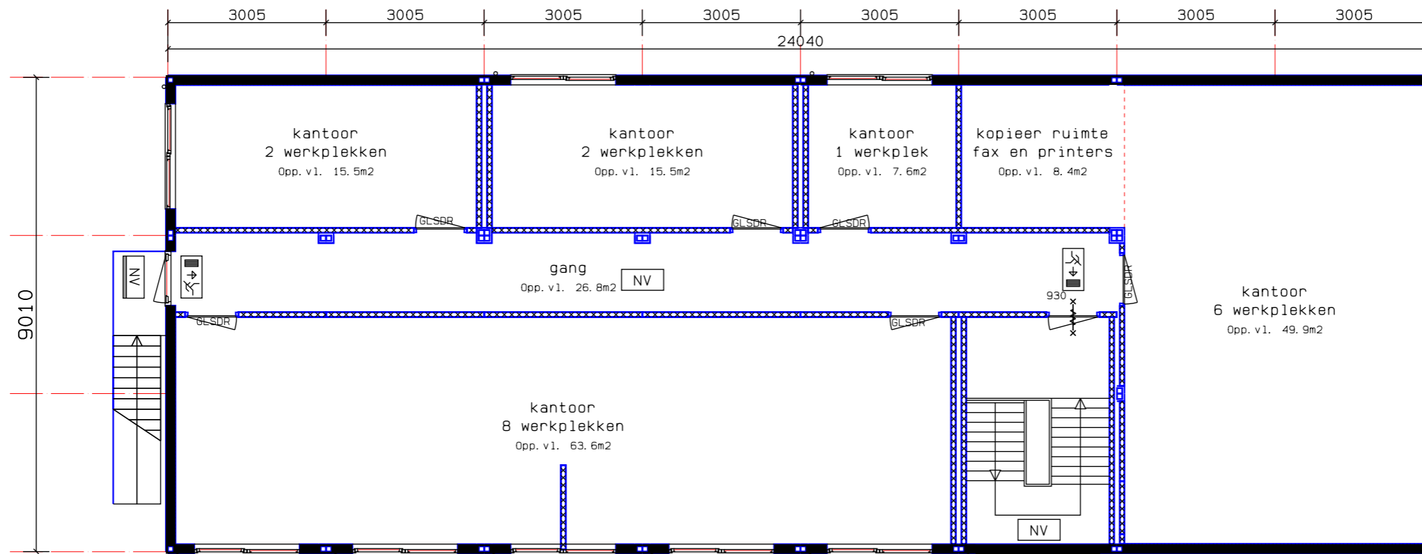
Plattegrond - 1e verdieping
